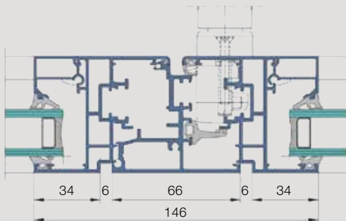
Fenster US-2: Horizontalschnitt mit Mittelpartie
