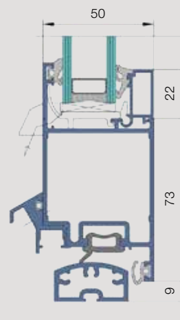
Tür US-2: Vertikalschnitt einwärts öffnend
