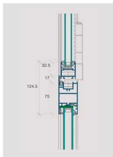
Brüstung (Festverglasung) mit Faltewand
