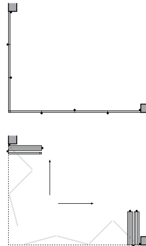
Pfostenlose Eckanlage 90°
