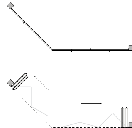
Pfostenlose Eckanlage 135°
