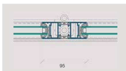
Mittelpartie mit Innenband
