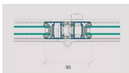
Mittelpartie mit Verschluss, einwärts öffnend
