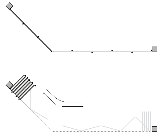
Pfostenlose Radiananlage 135°
